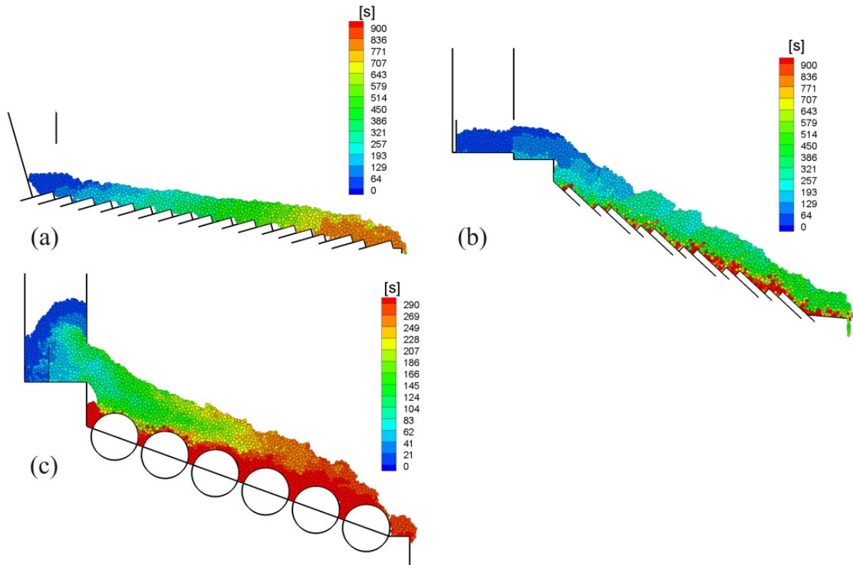
Partikelverweilzeit des Vorschubrostes (a), des Rückschubrostes (b) und des Walzenrostes (c)
