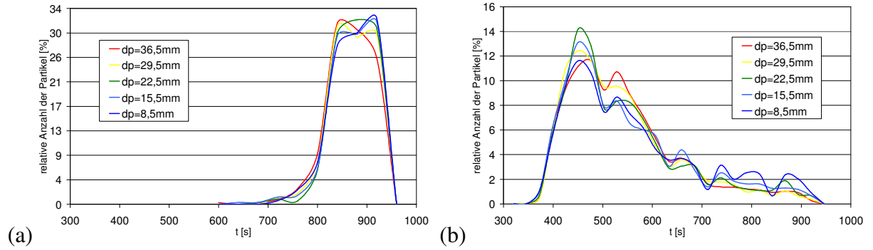
Verweilzeitverteilung der Partikelgrößenklassen des Vorschubrostes (a) und des Rückschubrostes (b)
