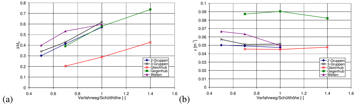
Vergleich der Bewegungsmuster mit 10 mm Kugeln: (a) Verbesserung des Mischungsstandes, (b) Mischungseffizienz
