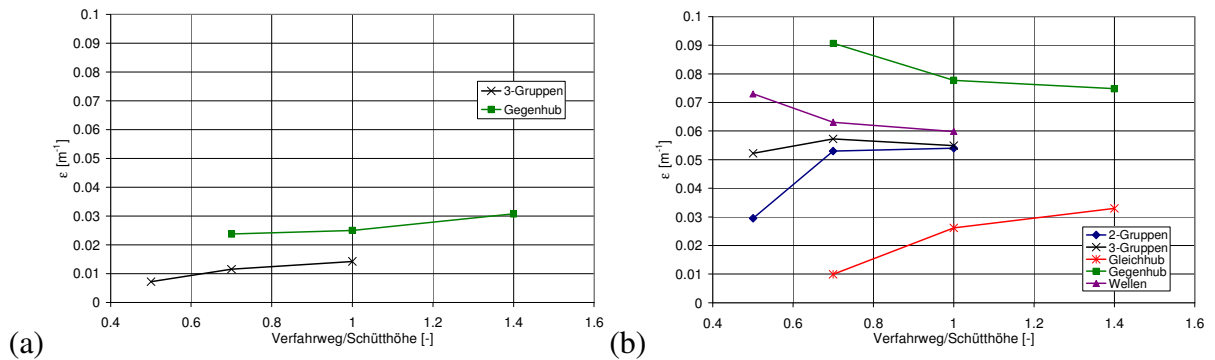
Mischungseffizienz für die Bewegungsmuster der Versuche mit (a) 5 mm Kugeln und (b) 20 mm Kugeln
