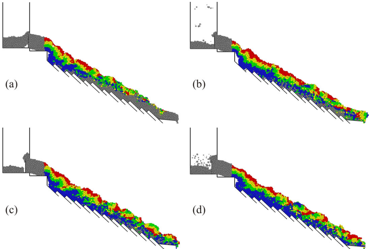
Momentaufnahme des Rückschubrostes nach (a) 250 s, (b) 500 s, (c) 750 s und (d) 1000 s
