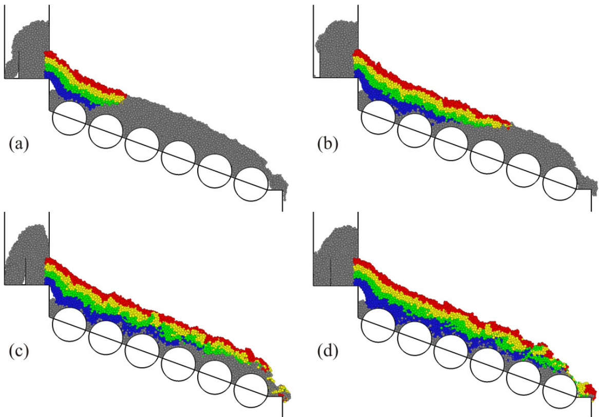
Momentaufnahme des Walzenrostes nach (a) 70 s, (b) 140 s, (c) 210 s und (d) 290 s
