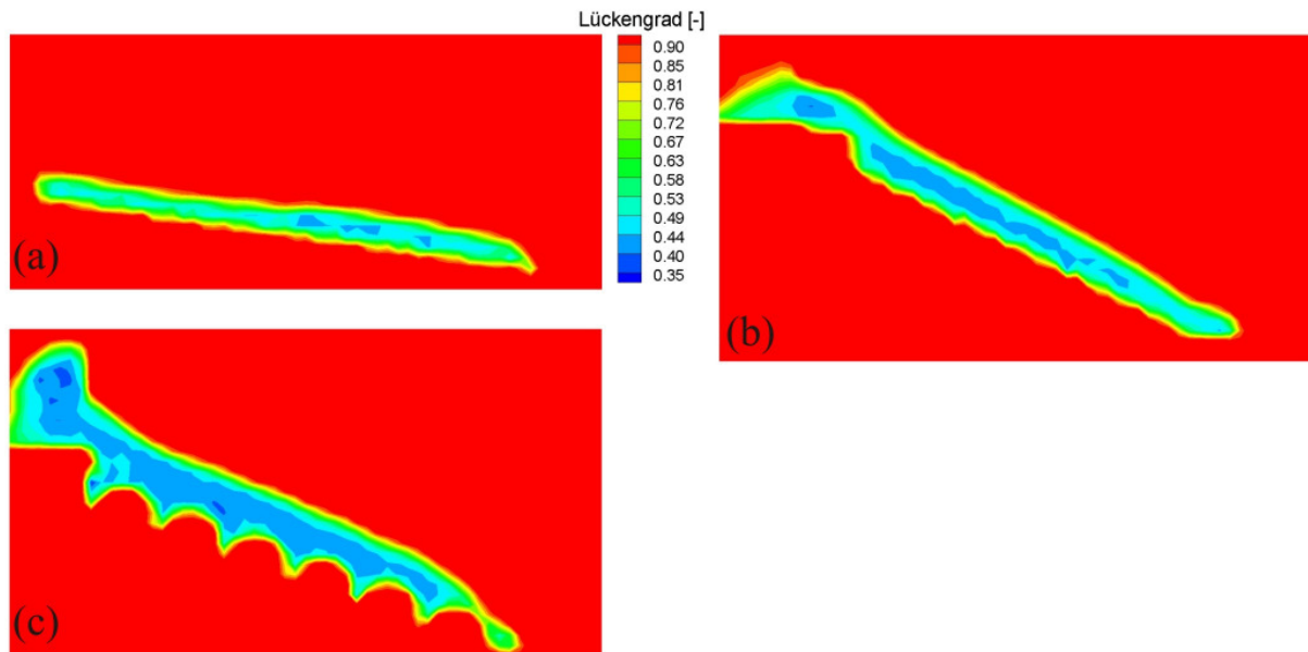
Lückengradverteilung für (a) Vorschub-, (b) Rückschub- und (c) Walzenrost
