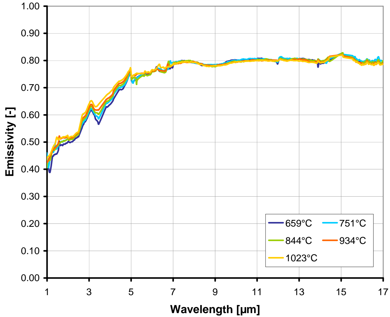
SiO 2 ; thermisch unbehandelt; SP1.25; 09.01.2007
